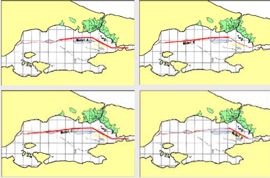
GRAFİK 5 JICA SENARYO DEPREMİ İÇİN FAY MODELLERİ (Kaynak: İBB, JICA, 2002)
